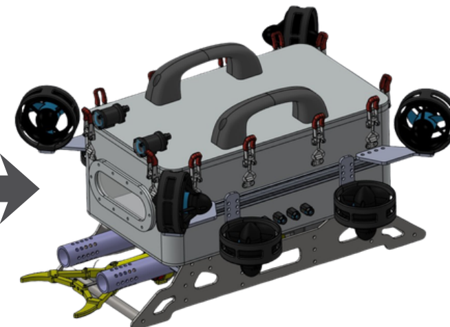
HAUV 2.0
